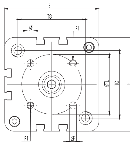
Ø32-40-50-63-80-100
