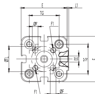
Ø20-25
