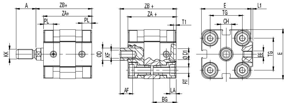
Ø32-40-50-63-80-100
