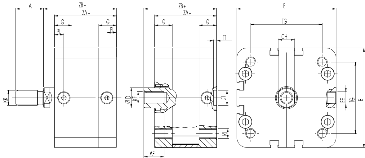
Ø32-40-50-63-80-100
